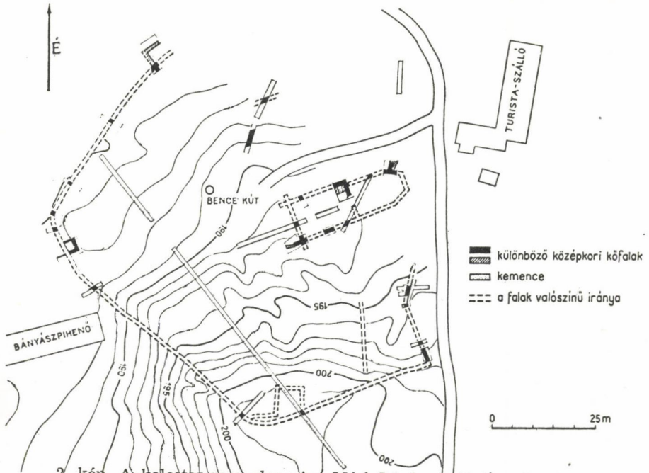
2. kép. A kolostor-rom alaprajza Méri István feltárása alapján
